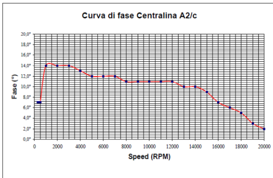
Curva di fase dell'accensione SELETTA A2/c Statore 2 Poli Ø 58.
